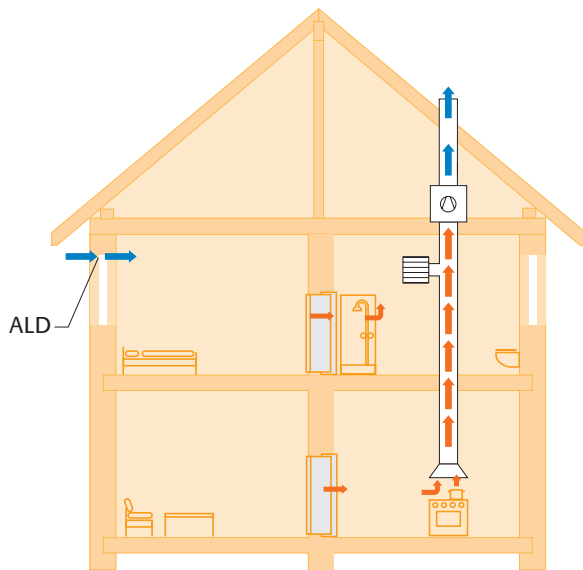
Abluftanlage mit Außenwand-Luftdurchlass (ALD)
